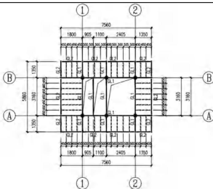
图 2-2 箱式变压器钢平台结构示意图
