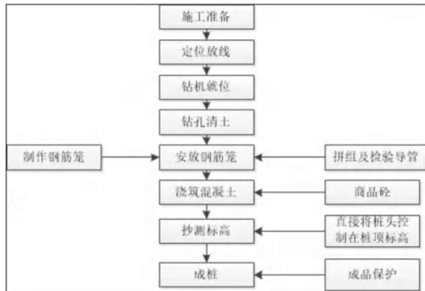
图 2-3 支架基础施工工艺流程图
