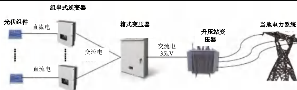
图 2-1 光伏发电过程示意图
