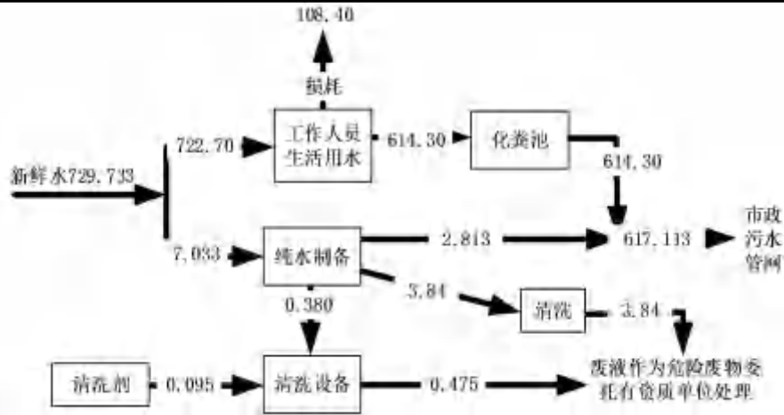
图 2-1 本项目水平衡图 单位: m³/a
