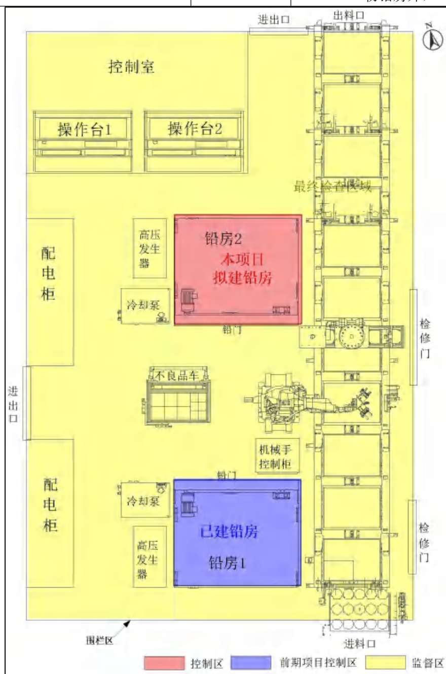
图 10-1 本项目自动化 X 射线探伤检测区域平面布局及分区图
