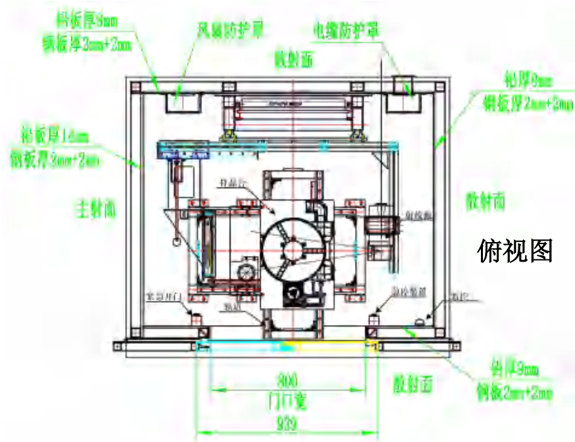
图 10-2 铅房屏蔽设计及结构示意图
