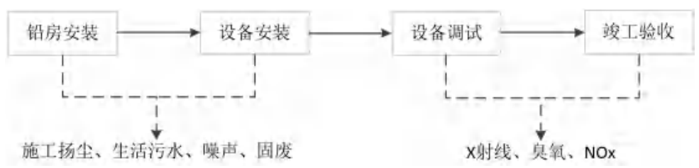
图 9-1 施工期工艺流程及产污环节图
